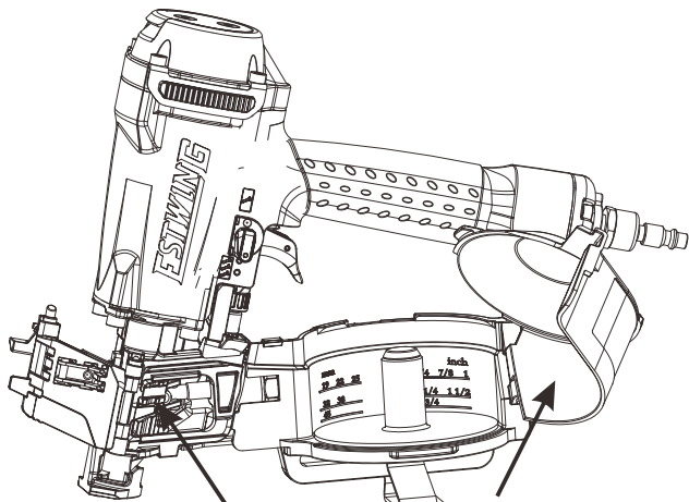
Chargeur (G) Couvercle du magasin (H)
